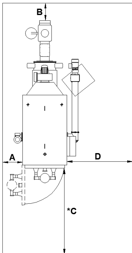
Anbefalede mindste afstande i fyrrummet
