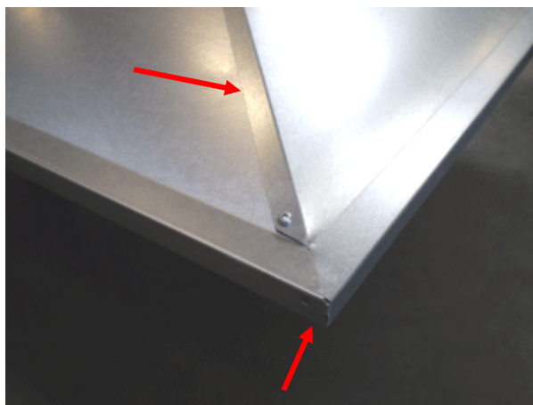
Hjørnesamling på låget
