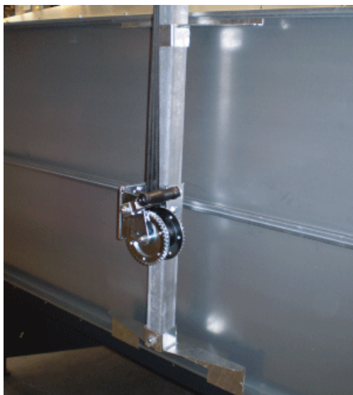
Søjle placeret i det nederste beslag
