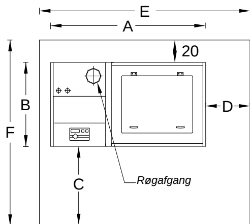
Fyrrum set fra oven - mål i cm.
